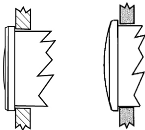
Elite Bezel Profile
